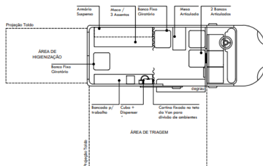
PLANTA BAIXA - CONSULTÓRIO NA RUA ESC. 1:50
